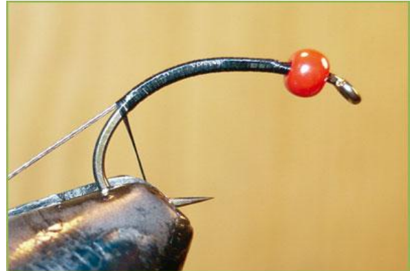
Etape 2 : fixer (en partant de contre la perle) à la courbure un rachis de plume de cou de coq (le fixer côté pointe).
